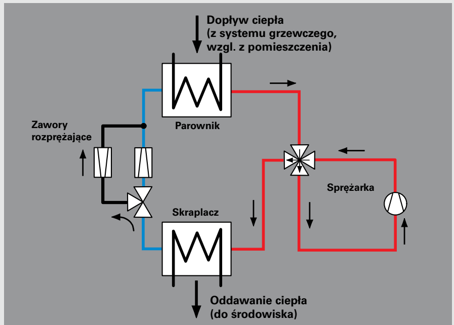
Rys. 2. Uproszczony schemat działania odwracalnej pompy ciepła w trybie chłodzenia
