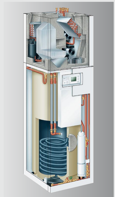
Rys. 4. Vitotres 343 – kompaktowa centrala dla domów pasywnych – pompa ciepła kombinowana z systemem odzyskowej wentylacji pomieszczeń i pojemnościowym podgrzewaczem c.w.u.
